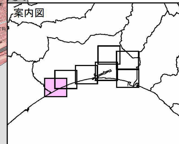
想定津波波源域
